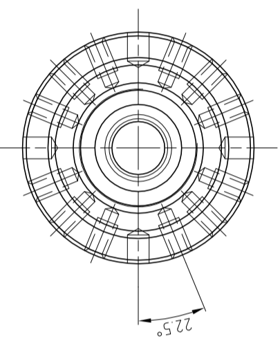
Ansicht "A"
